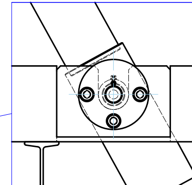
Sistema de articulación inferior de cilindro B ( 1 : 10 )
